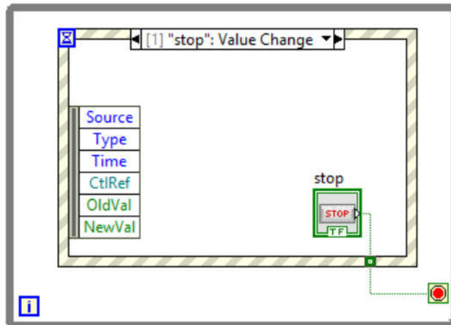
Sl. 2.7.4. Ispravan način zaustavljanja While petlje koja ima Event strukturu
