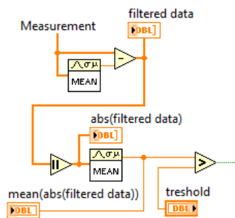
Sl. 4.8.4: Procena anvelope analognog signala sa mikrofona ai0
