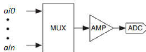
Sl. 4.3.3. Multipleksiranja analognih kanala – AMP je pojačavač, ADC je analogno-digitalni konvertor
