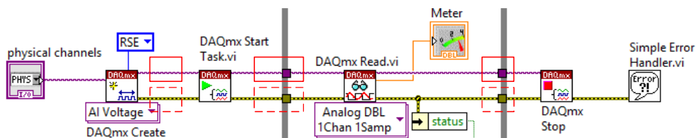
Sl. 4.2.10. Punom linijom su zaokružene task linije, a isprekidanom error linije
