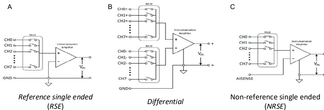
Sl. 4.10. Različite konfiguracije za povezivanje ulaznih signala na A/D karticu
