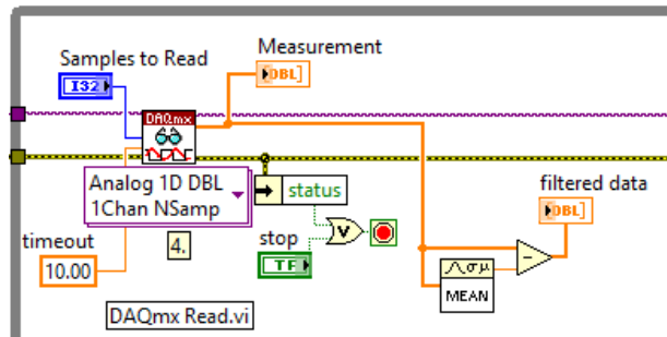
Sl. 4.8.2. Otklanjanje jednosmerne komponente
