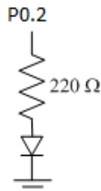
Sl. 4.5.2. Veza linije 2 digitalnog kanala 0 (P0.2) i LED diode
