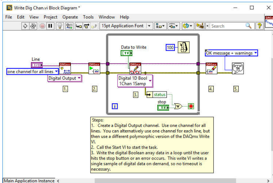
Sl. 4.5.1. Block Diagram aplikacije Write Dig Chan.vi
