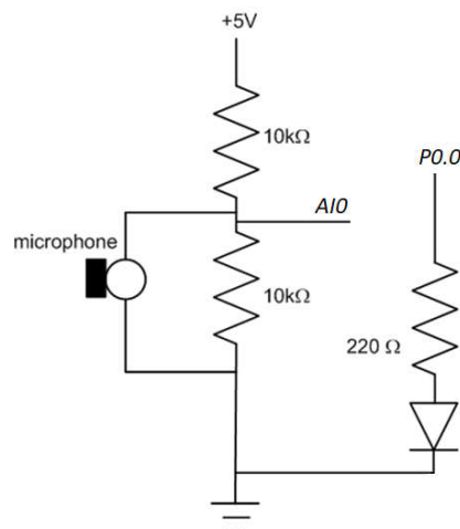
Sl. 4.8.1. Šema povezivanja
