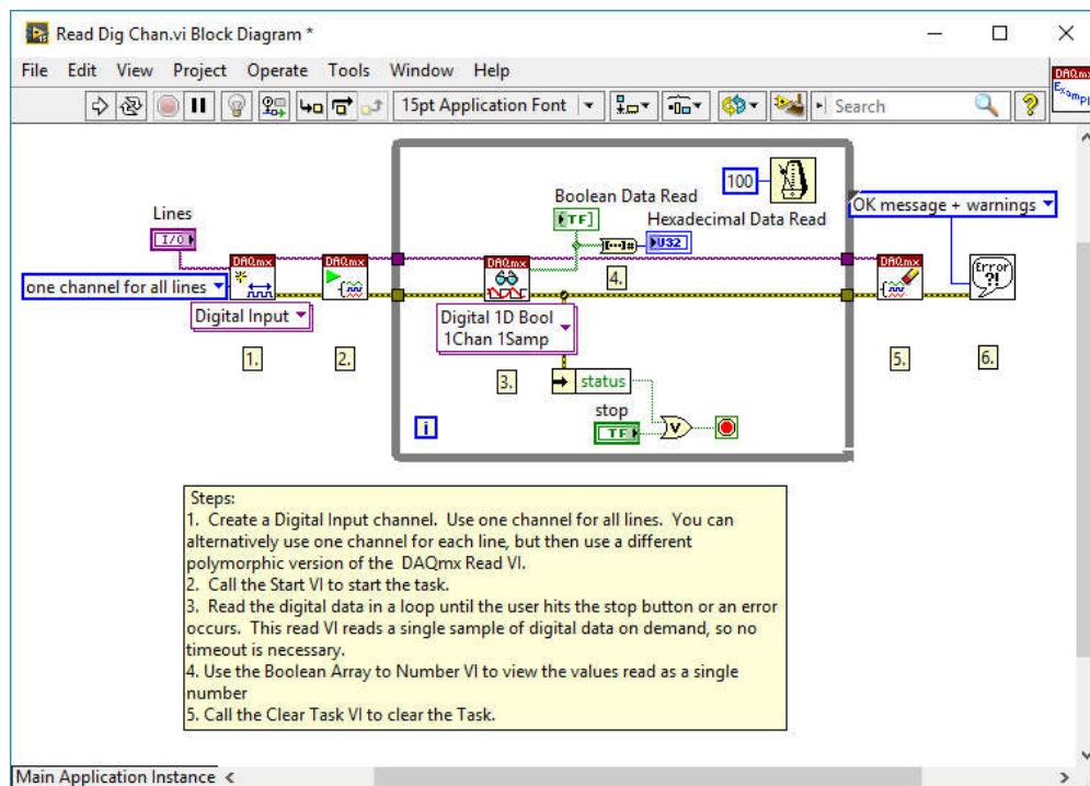
Sl. 4.4.2. Block Diagram aplikacije Read Dig Chan.vi
