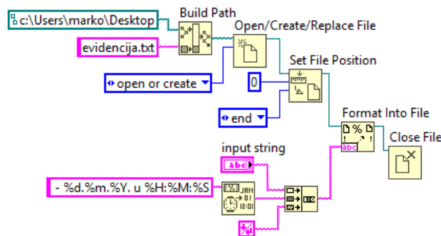
Sl. 8.18. Kod za VI “Loguj pocetak_kraj rada”.
